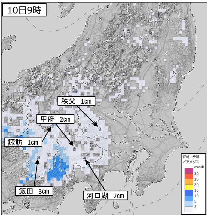
3時間降雪量 (解析値とアメダス観測値)
